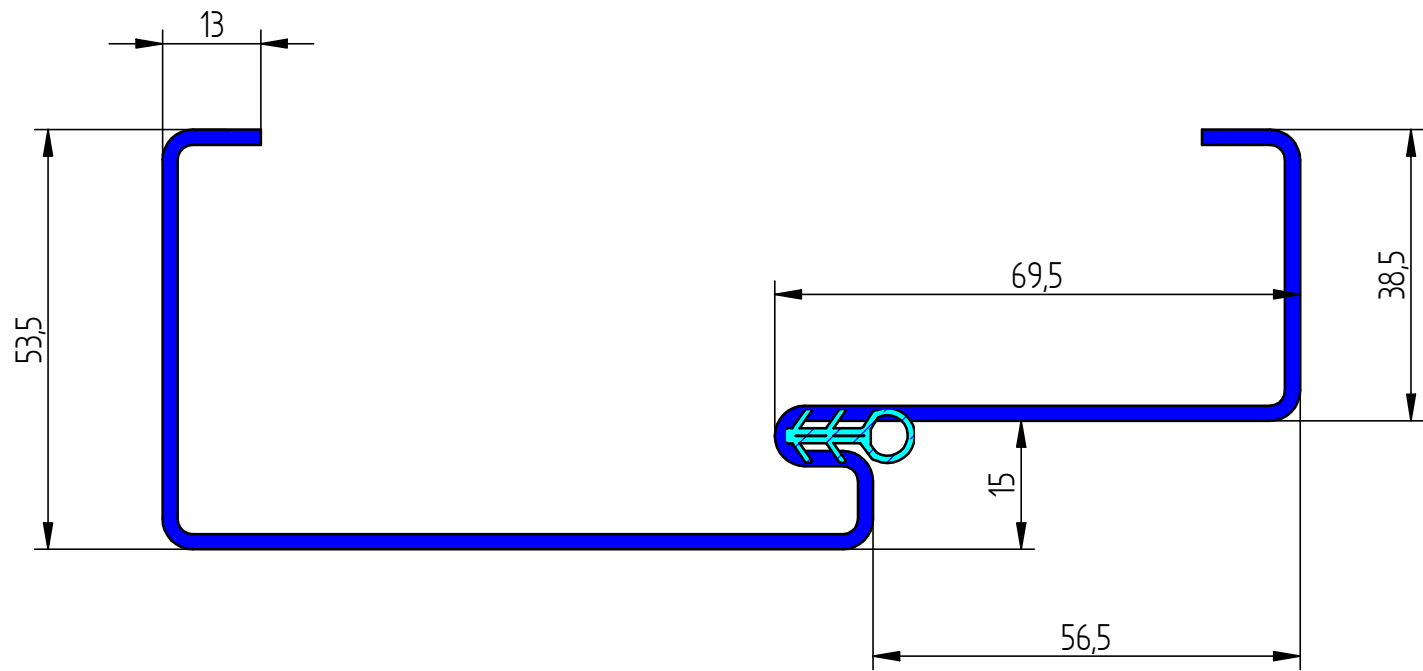
טיפוס 97H פלץ אחד+גומי אטימה
