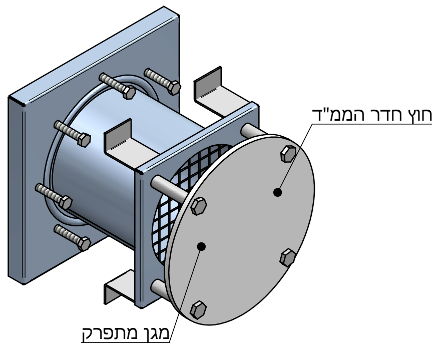
צינור 8" לממ"ד-קיר חיצוני לבנייה מתועשת
